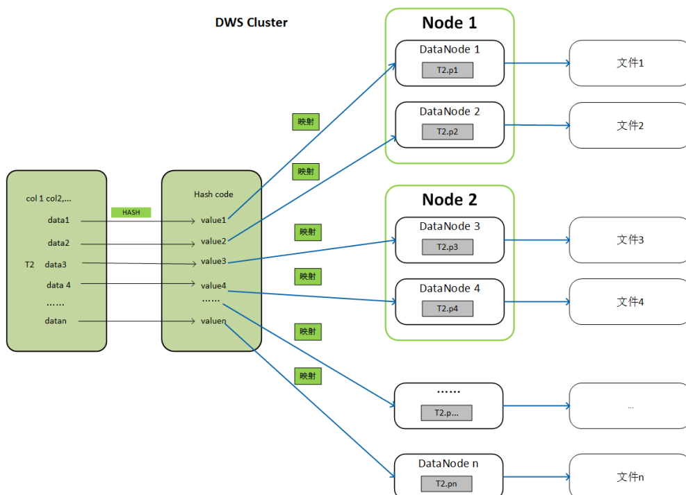
图 9-1 Hash 分布原理
